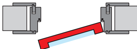
ZPŮSOB MONTÁŽE MATNÉHO SKLA (KŘÍDLO PRAVÉ - MATNÁ ČÁST SMĚREM K POZORUJÍCÍMU) SPÔSOB MONTÁŽE MATNÉHO SKLA (KŘÍDLO PRAVÉ - MATNÁ ČÁST SMEROM KU KLIENTOVI)
