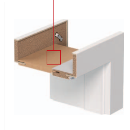
ŘEZ ZÁRUBNĚ S REGULAČNÍM PANEĽEM REZ ZÁRUBNE S REGULAČNOM PANEĽOM
